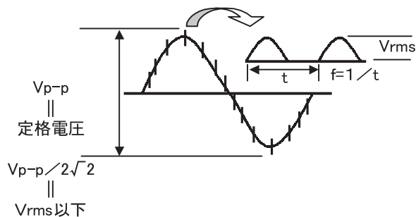
直流平滑時の高周波リプル例
