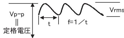
直流平滑時の高周波リプル例
