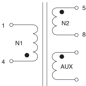
外形尺寸和电原理图
