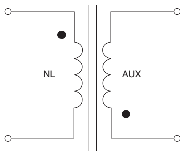
外形尺寸和电原理图
