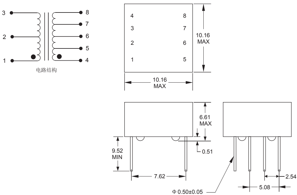
图1 结构G外形尺寸和电原理图
