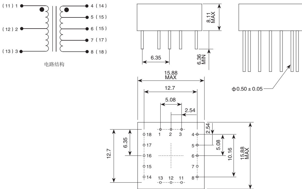
图1 结构K外形尺寸和电原理图
